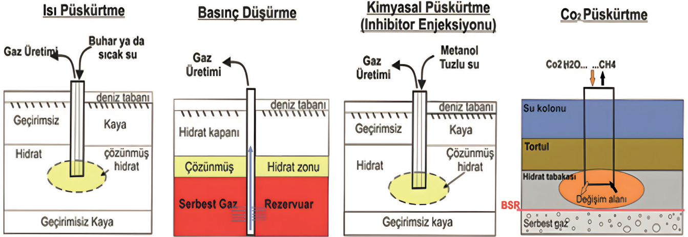
Şekil 5. Gaz hidratlardan doğal gaz elde etmek için uygulanabilecek üretim yöntemleri. Isı püskürtme, Basınç düşürme, kimyasal püskürtme ve CO2 değişimi, her biri benzersiz faydalar ve zorluklar sunar. (Şekil: Çifci vd., baskıda).
