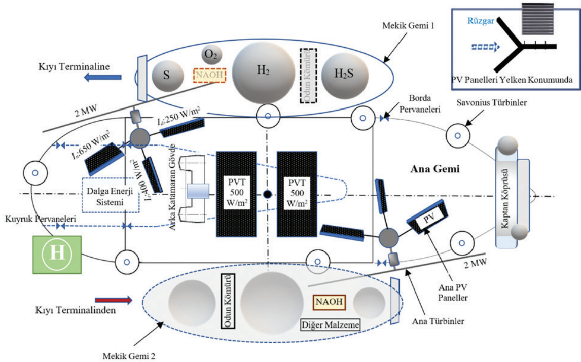
Şekil 4: Karadeniz Ana Hidrojen Gemisi, H/S Sinop ©B. Kılıkş
