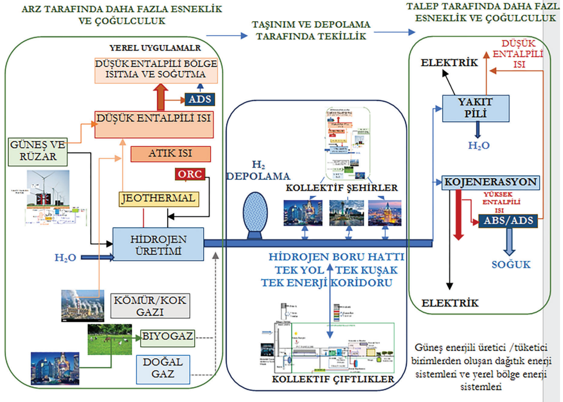
Şekil 18. KYG'de Olası Nihai Çözüm: Tek Bir Yeşil Enerji Buluşmasında Tek Kuşak, Tek Enerji Koridoru
