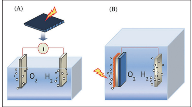
Şekil 10. Fotovoltaik Entegre Edilmiş Elektroliz ile Su Ayrıştırma Sistemi A) Fotovoltaik Sistem ve Dış Elektrolizör B) Fotovoltaik Entegre Elektroliz Hücresi
