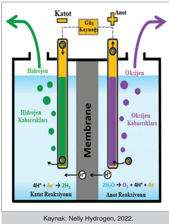
Şekil 5. Alkali Elektroliz Hücresi
