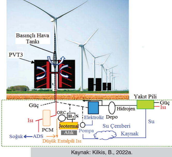
Şekil 16. Yeraltı ve Yerüstü Yenilenebilir Enerji Kaynaklarını Tümluştiren Kompozit Yenilenebilir Enerji Sistemleri
