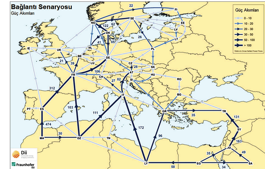
Şekil 8. Bağlantı Senaryosu
