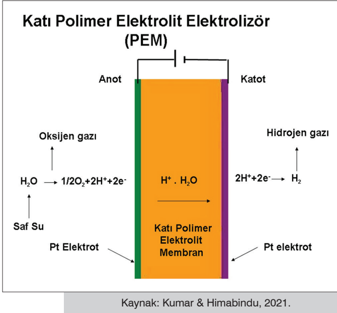
Şekil 6. PEM Elektrolizör
